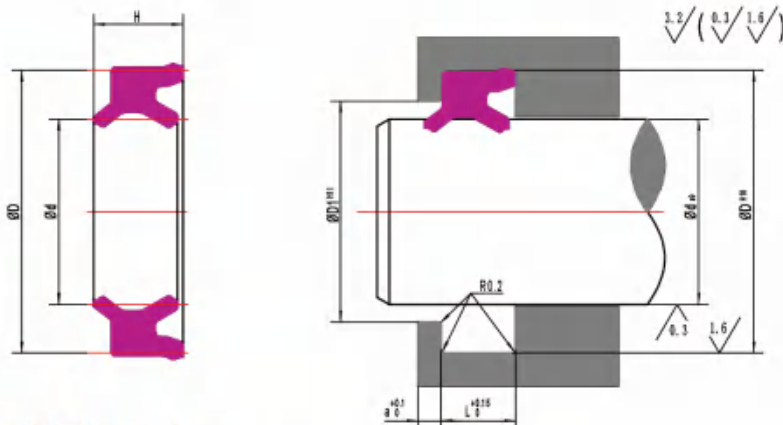
PRM型标准规格表 (单位: mm) PRM Standard specification sheet (Unit: mm)
