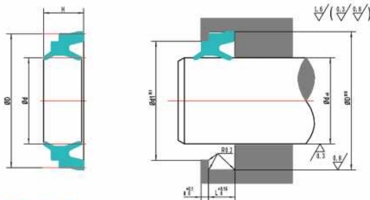
PRL型标准规格表 (单位: mm) PRL Standard specification sheet (Unit: mm)
