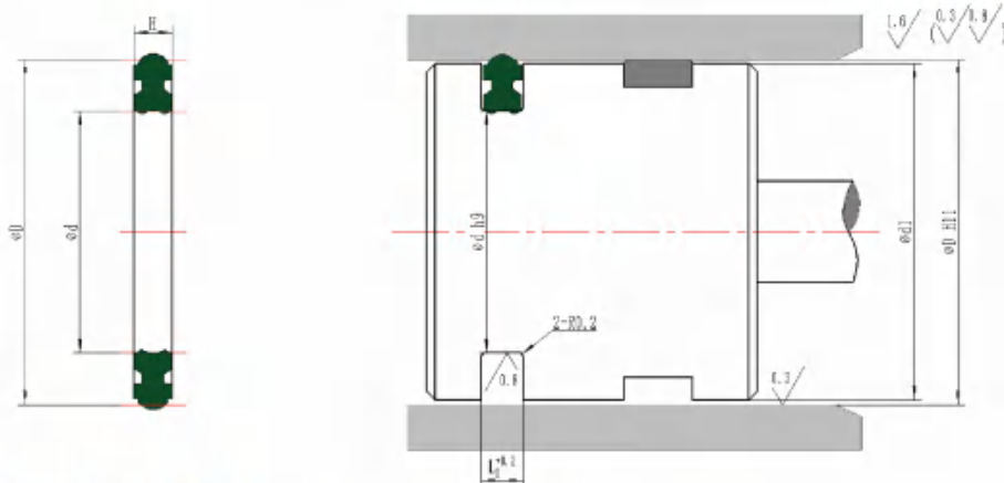
PPA型标准规格表 (单位: mm) PPA Standard specification sheet (Unit: mm)
