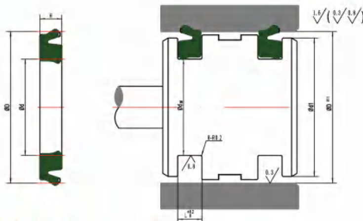
PPS型标准规格表 (单位: mm) PPS Standard specification sheet (Unit: mm)
