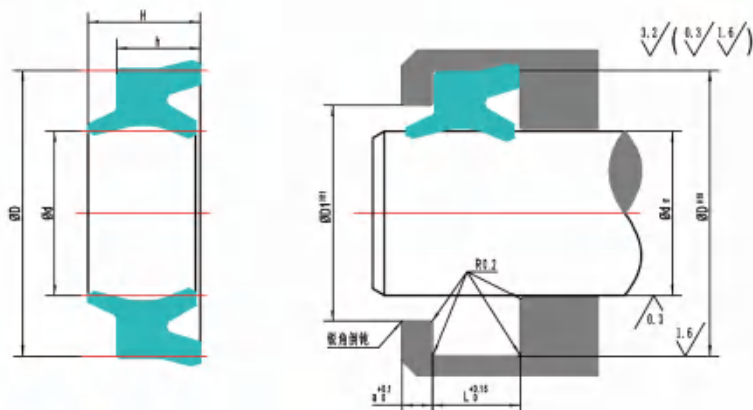
PRD型标准规格表 (单位: mm) PRD Standard specification sheet (Unit: mm)
